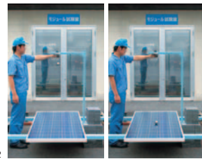
1) Comprobación de la capacidad de carga estática 2) Comprobación de la resistencia al impacto
